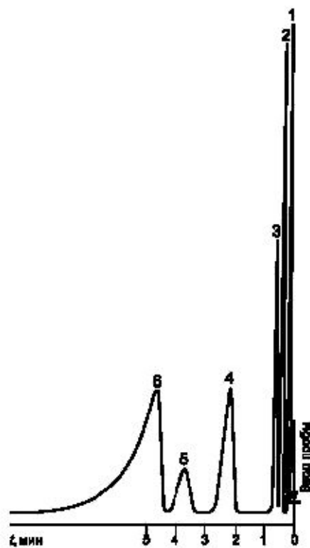
Типовая хроматограмма растворителя марки 646
