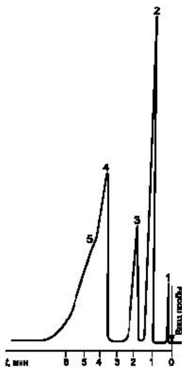
Типовая хроматограмма растворителя марки 647
