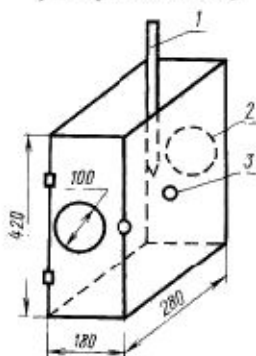
1 — пипетка; 2 — смотровое стекло; 3 — отверстие для зажима
